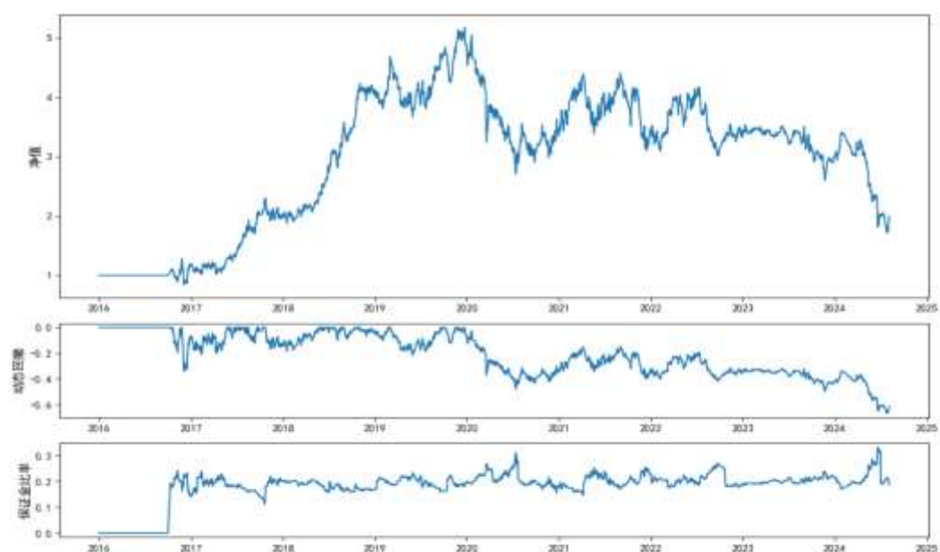
图 2：成交量偏度测试结果
