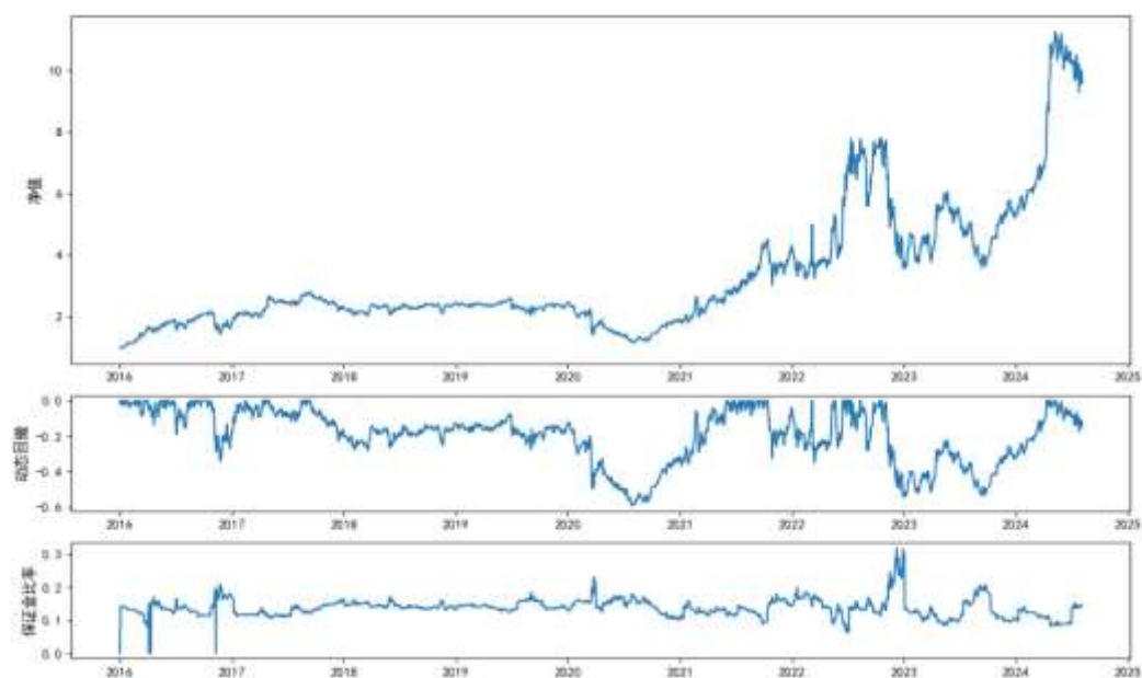
图 6：收益率峰度与偏度比值测试结果
