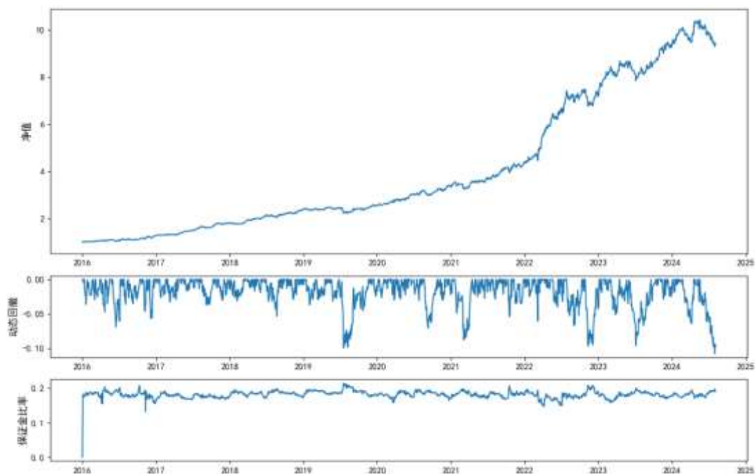
图 7：动量组合测试结果
