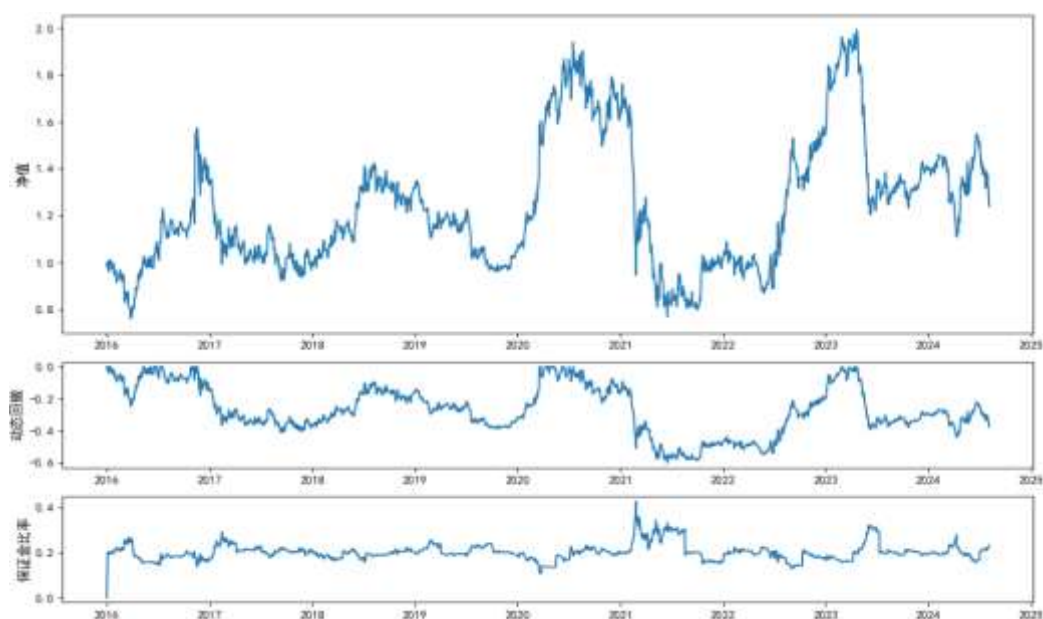
图 1：成交量峰度测试结果
