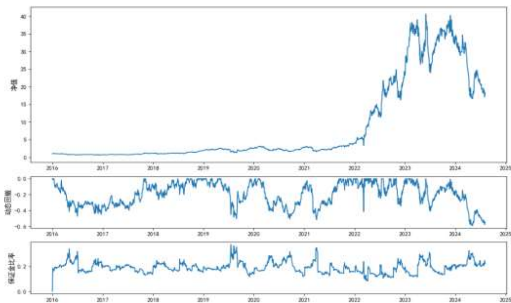
图 5：收益率偏度测试结果
