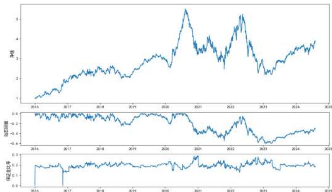
图 3：成交量峰度与偏度比值测试结果
